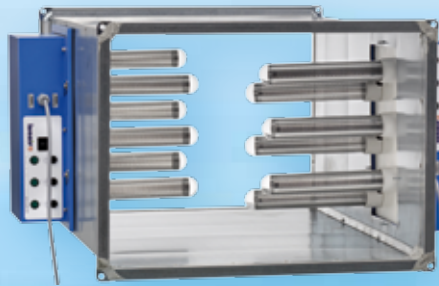
| Installation avec des cadres inox poudrés dans la canalisation
